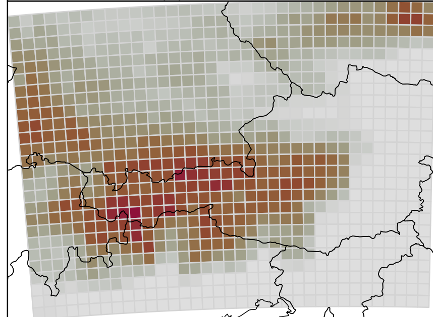
(d) Exceedance
