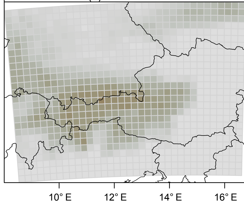
(d) Exceedance
