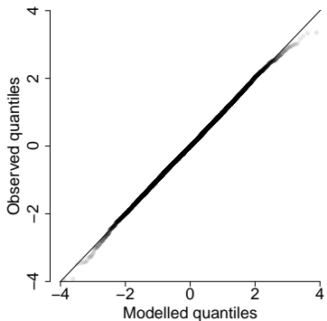
(d) quantile-quantile plot
